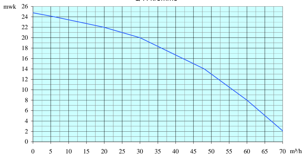
Q-H kromme
