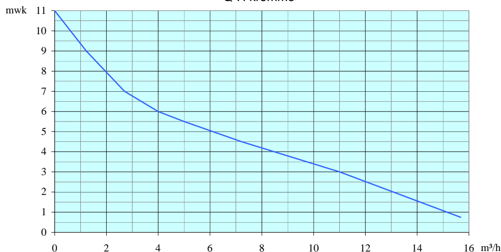
Q-H kromme
