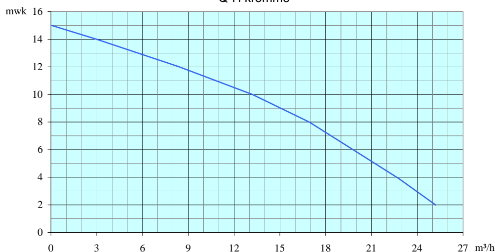
Q-H kromme
